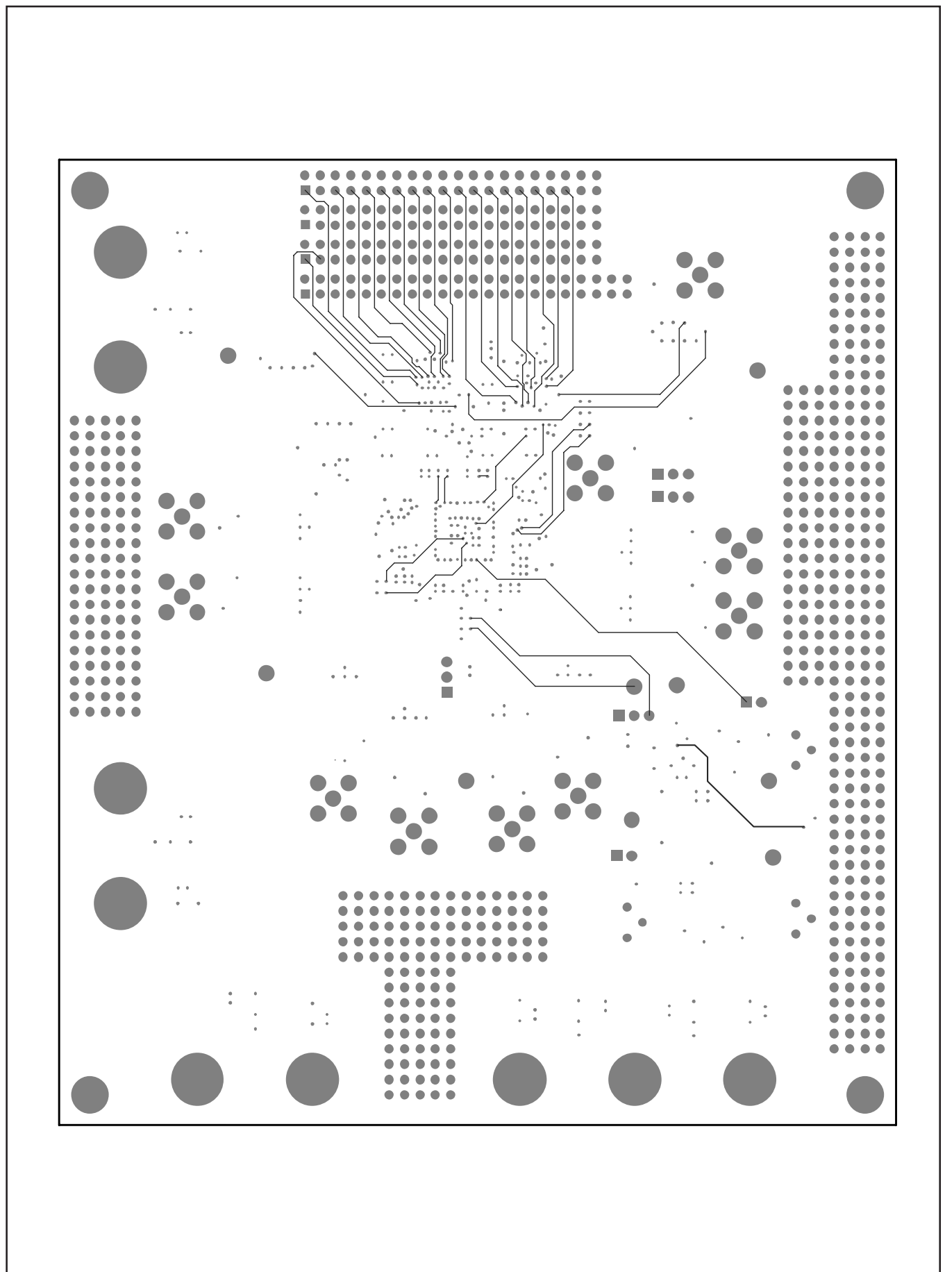
FIGURE 8. EVM Layer 3: Inner Layer I.
